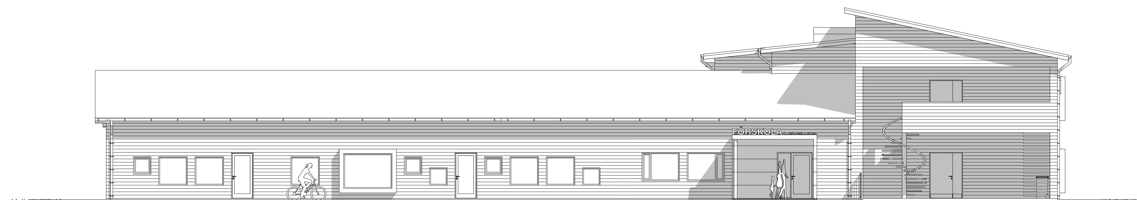
FASAD MOT ANGÖRINGSSIDAN, SKALA 1:100
