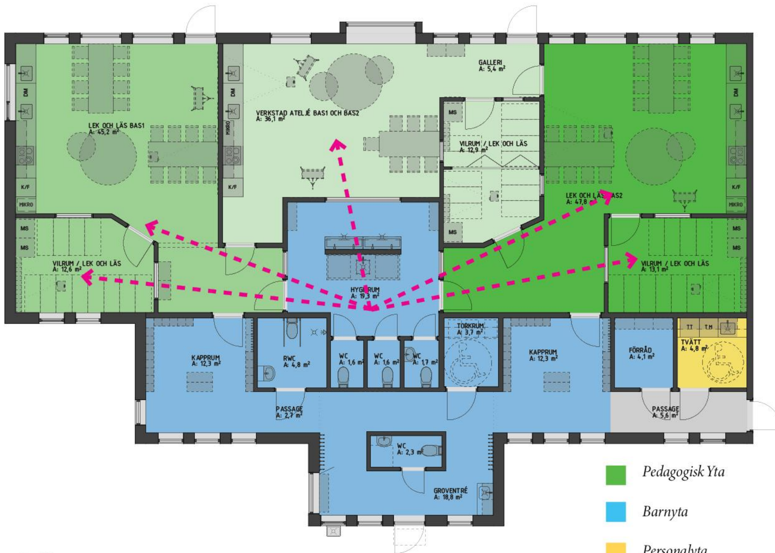
Typplan över en enhet med två baser.
